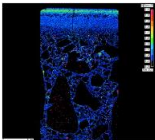
写真 9 硫黄分布
