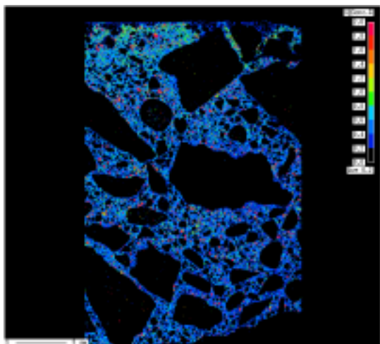
写真 9 硫黄分布
