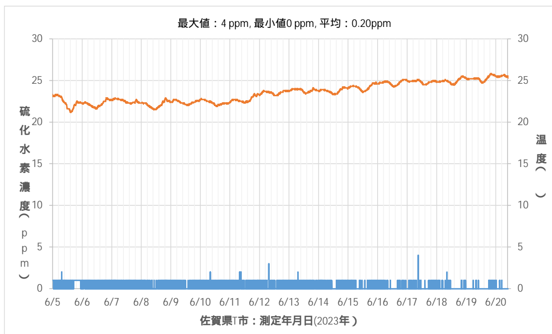
図 2 硫化水素濃度連続測定結果 (2023年6月5日~2023年6月20日)
