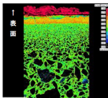
図－2 硫黄の存在形態分布例
