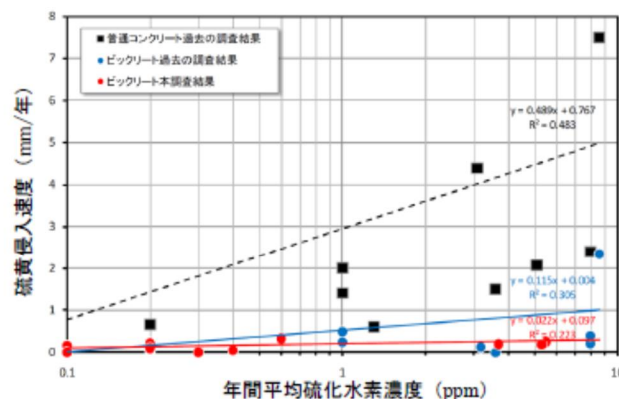
図-5 硫化水素濃度と硫酸侵入深さの関係 4)
