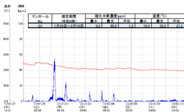
図-4 硫化水素濃度測定結果一例
