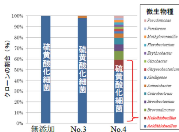
図-3 微生物種の同定結果
