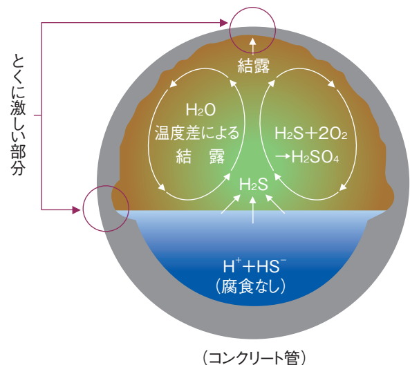
●下水管の腐食の原理
